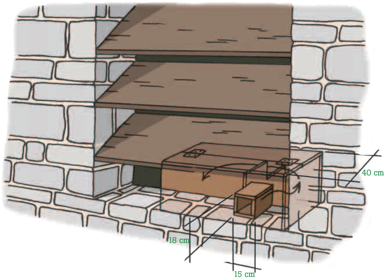
Schéma d'un nichoir avec galerie d'accès simple
