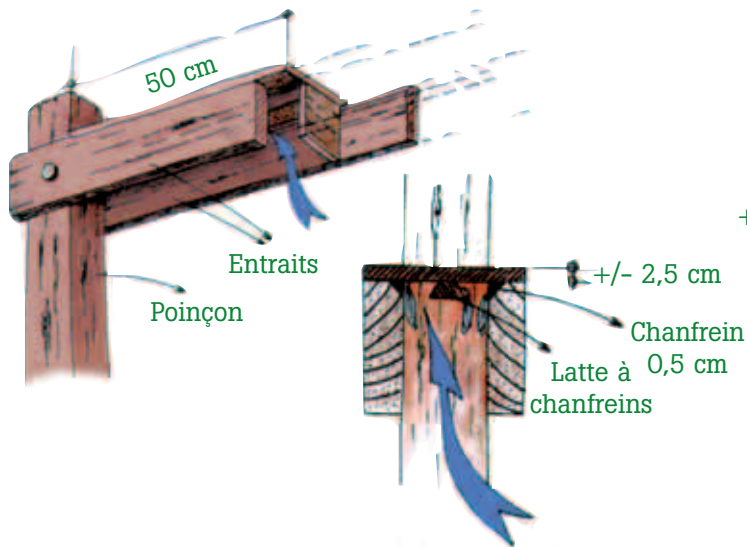
Construction entre entrails parallèles
