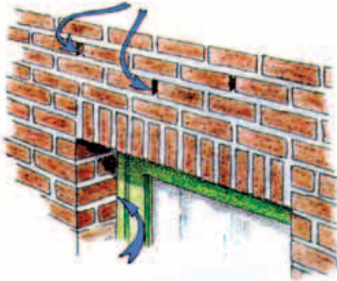
Accès par un joint resté ouvert dans le mur de parement
