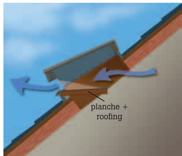
Avec planche d'envol
