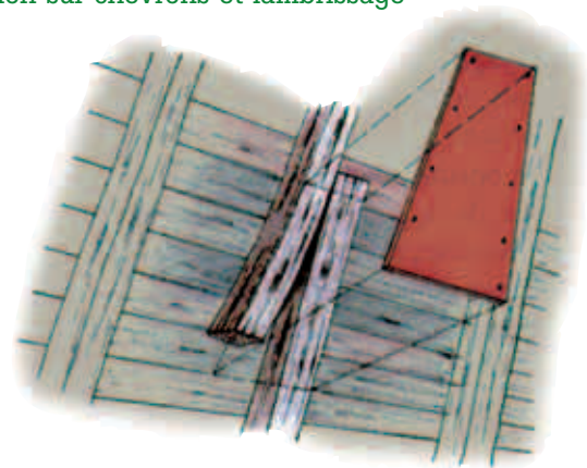
Construction sur chevrons et lambrissage
