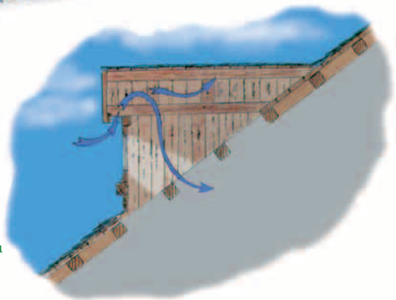
Ouverture pratiquée sur le fronton
