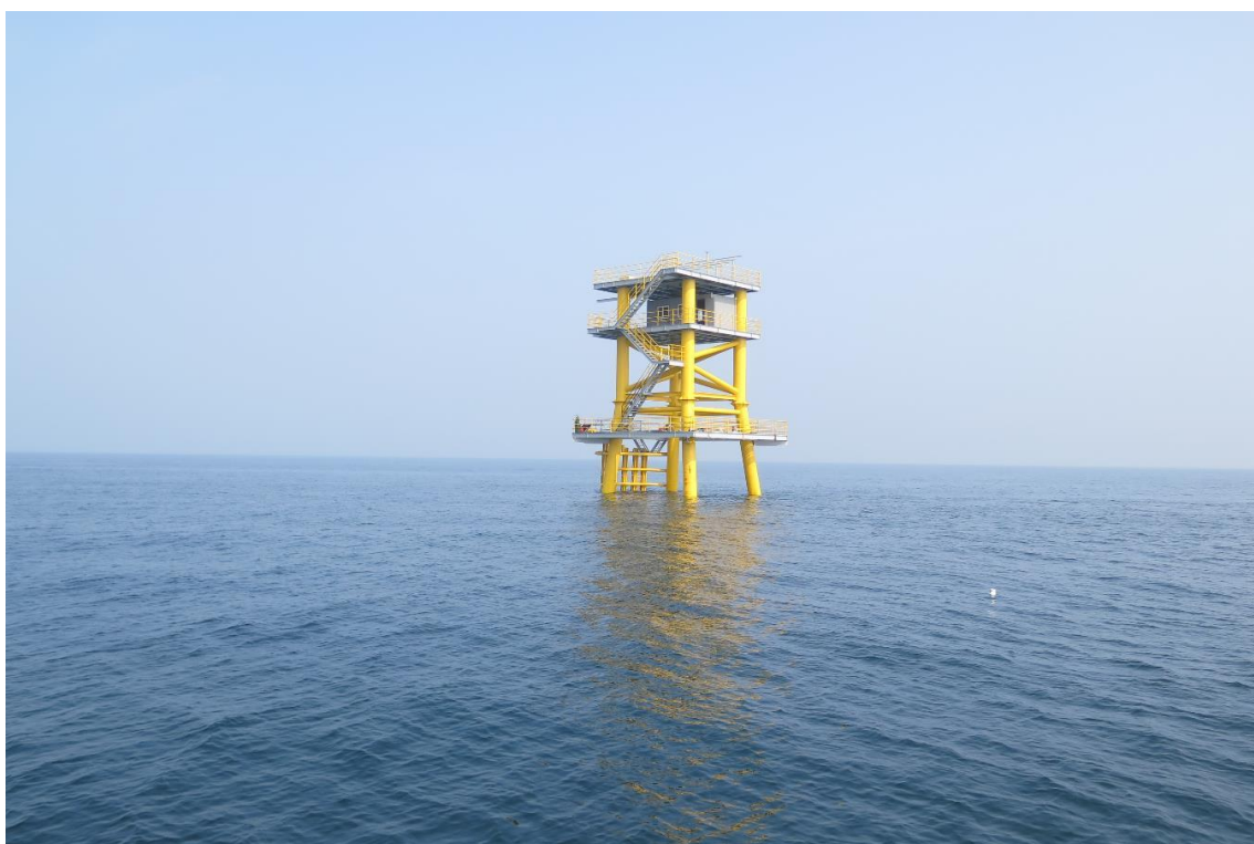
KEPCO : Plateforme au large de Gunsan en Corée du Sud
