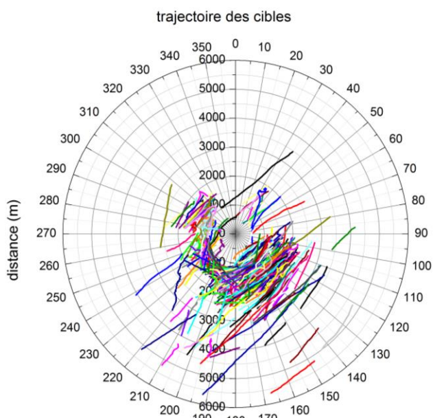
Figure 5: trajectoire des pistes ayant une durée de vol > 45s durant la journée du 13-11-2017
