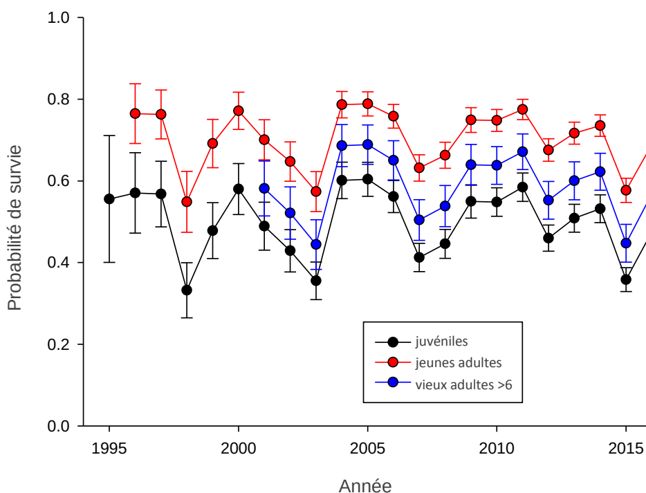
Fig. 5. Probabilités de survie annuelle ( \pm SE) en fonction de trois classes d'âge (juvéniles (en noir), jeunes adultes (entre 2 et 6 ans, en rouge) et vieux adultes (entre 7 et 14 ans, en bleu) avec un effet additif sur le temps (issu du modèle M8).
