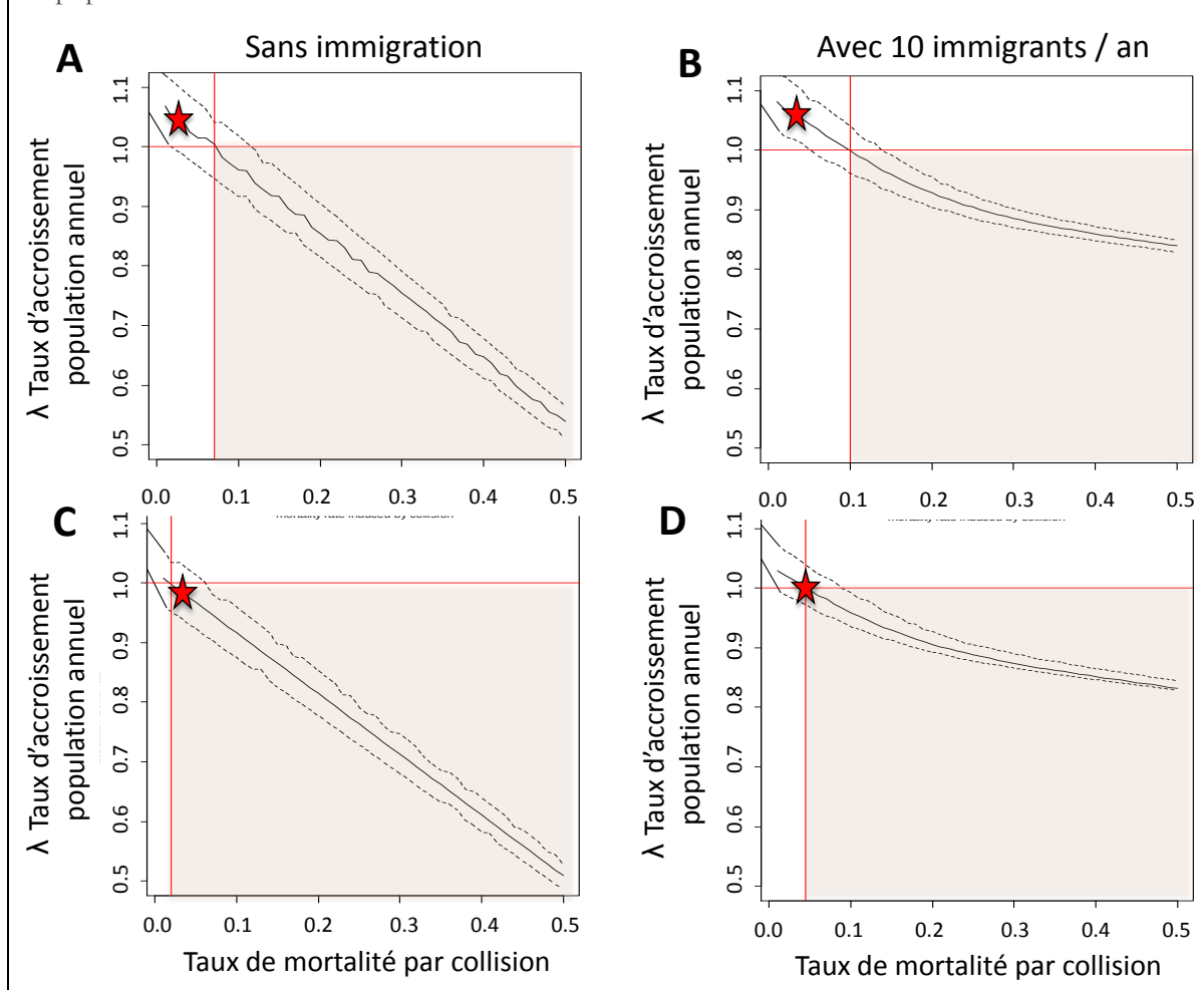
Fig. 7. Variation du taux de croissance inter-annuel \lambda de la population de faucons crécerelletes, en fonction du taux de mortalité induit par les collisions avec les éoliennes. à gauche en l'absence d'immigration, à droite avec 10 immigrants par an ; A et B : avec une alternance équilibrée entre bonnes et mauvaises années ; C et D : avec 75% de mauvaises années, dues à une dégradation des conditions d'hivernage. Les lignes rouges indiquent le seuil de mortalité au-delà duquel la population décline ( \lambda < 1 , zone grisée). L'étoile rouge indique le taux actuel de mortalité par collision et le taux actuel de croissance de population.
