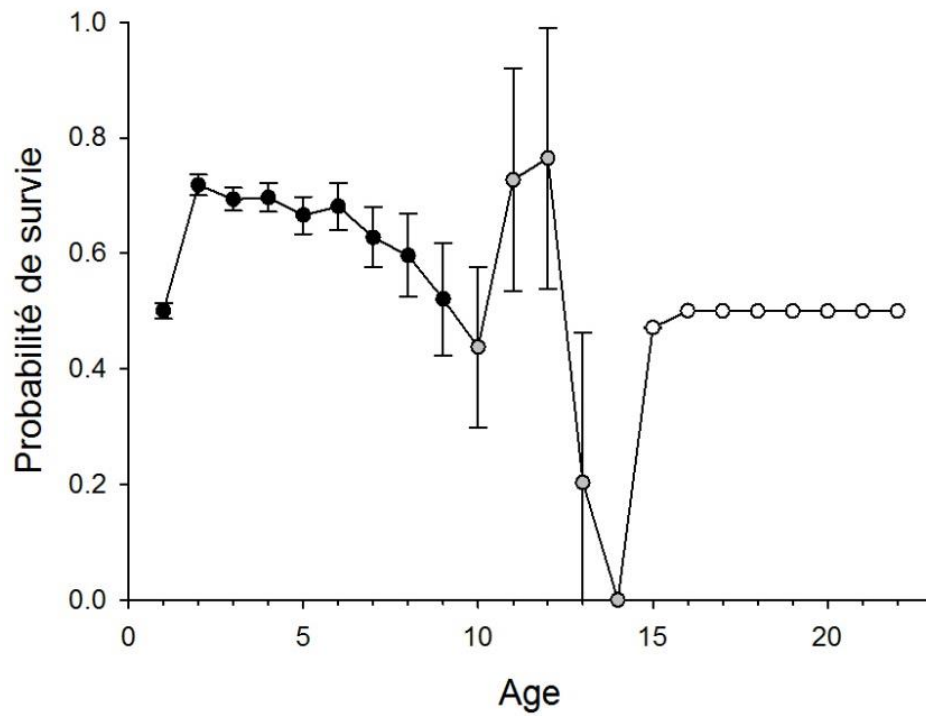
Fig. B.1 : probabilité de survie ( \pm SE) en fonction de l'âge des individus (issu du modèle M1). A partir de 10 ans, les estimations ne reposent plus que sur une vingtaine d'individus (points gris) et sur aucun individu à partir de 15 ans (points blancs).
