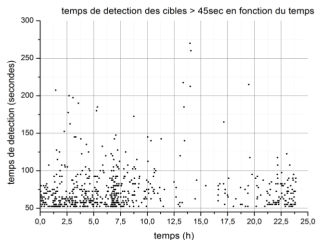
Figure 6: pistes ayant une durée de détection > 45 secondes durant la journée du 13-11-2017
