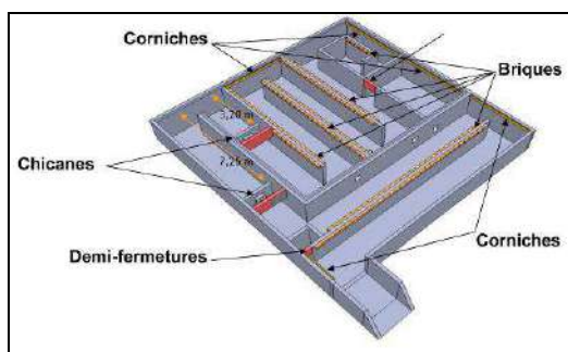
Exemple du gîte de substitution réalisé en forêt de Belles Forêts dans le cadre de la construction de la deuxième phase de la LGV Est européenne - (Source : RFF/Cpepesc Lorraine)
