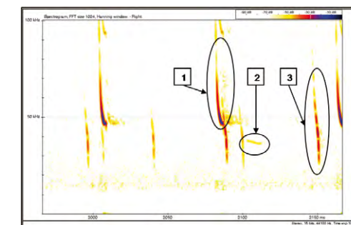
Le sonogramme permet de représenter graphiquement (fréquence en fonction du temps) les ultrasons des chauves-souris qui ont été enregistrés sur le terrain. C'est à partir de ce graphique que peuvent être identifiées les différentes espèces contactées lors d'un inventaire. Sur le sonogramme présenté, trois espèces peuvent être distinguées :
